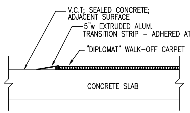
2 CARPET TRANSITION DETAIL A1.05 SCALE: N.T.S.
