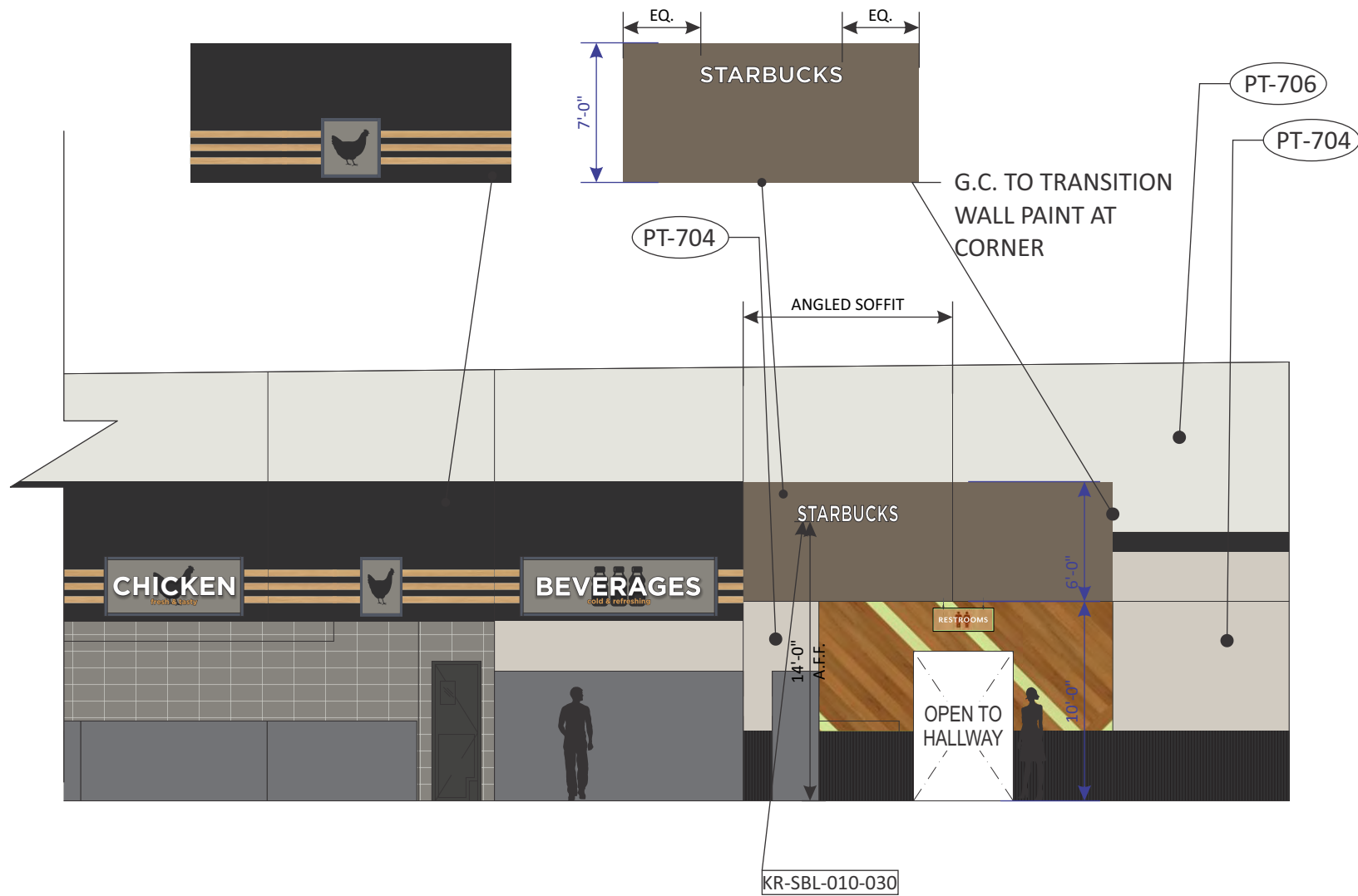
ELEVATION F SCALE: 1/8" = 1'- 0"
